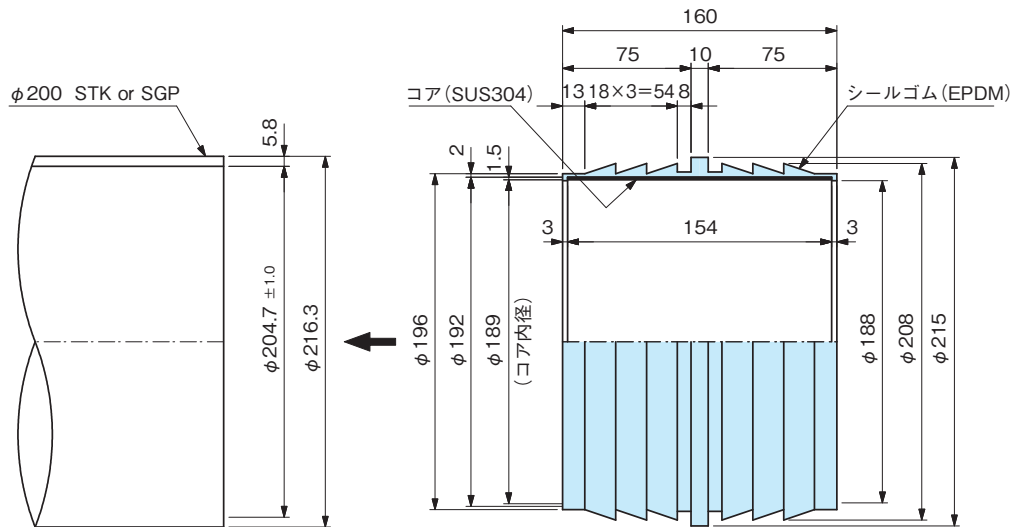
注 φ200 鋼管 STK or SGP t=5.8 mmに対応
